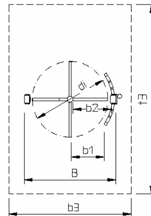
Kentaur - 90°, ochrana pred vplyvom prostredia – strieška s fasciou a odpadom
