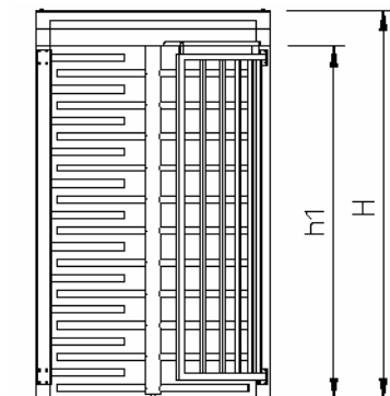
Kentaur - 180°, ohradený z boku oceľovými tyčami.
