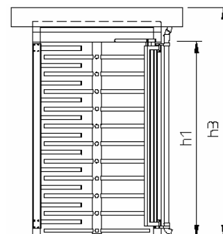
Kentaur - 90°, ochrana pred vplyvom prostredia – strieška s fasciou a odpadom
